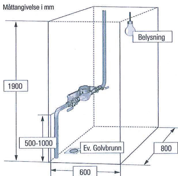
Exempel på godkänd mätarplats
